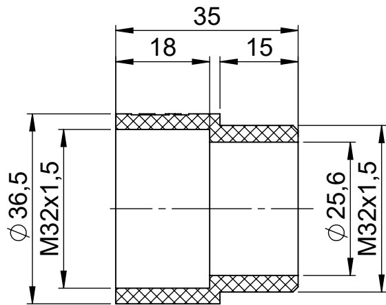
SCHNITT A-A
