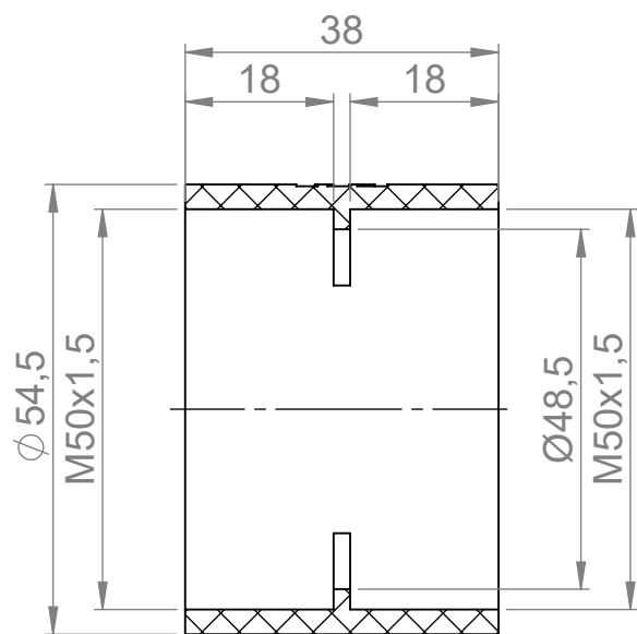
SCHNITT A-A
