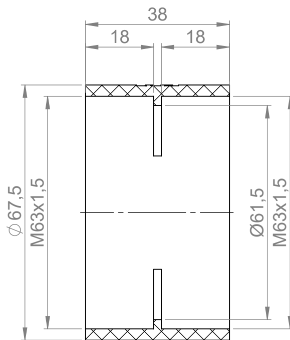
SCHNITT A-A
