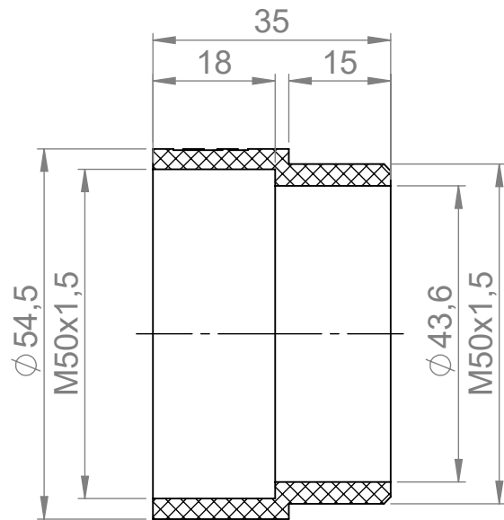
SCHNITT A-A
