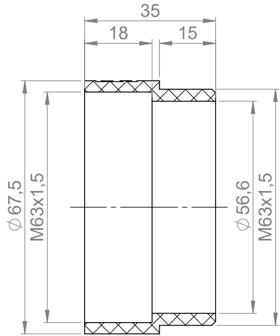
SCHNITT A-A
