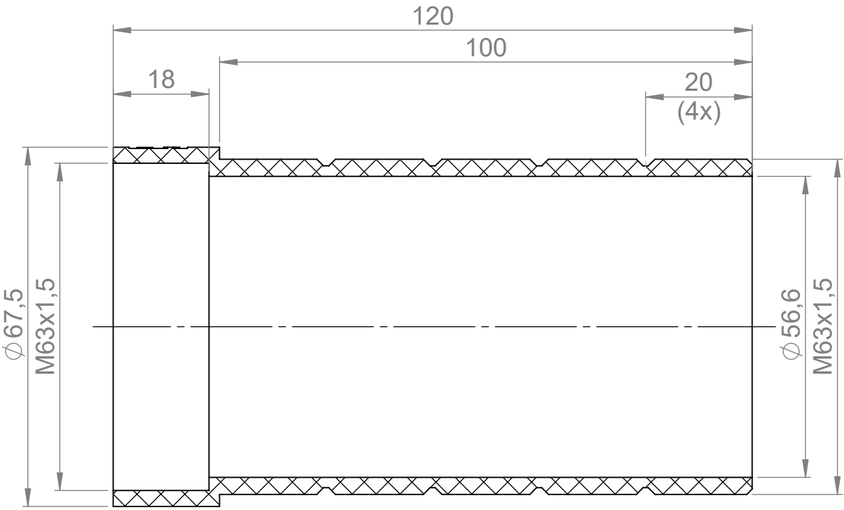
SCHNITT A-A
