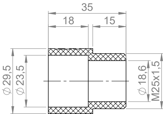
SCHNITT A-A
